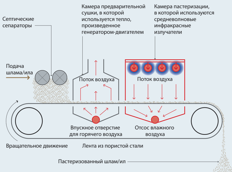
Рисунок 6: схема работы установки для гранулирования шлама/ила LaDePa
