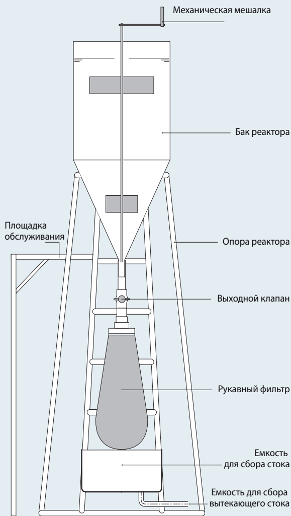
Рисунок 7: Схема реактора для производства струвита, оснащенного механической мешалкой и рукавным фильтром
