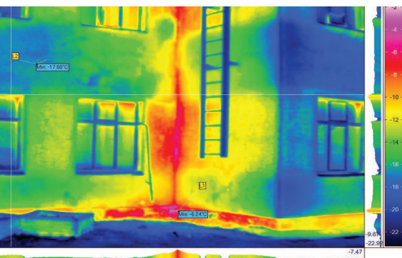
Ховд аймгийн сургуулийн барилгын дулаан хэмжилт
